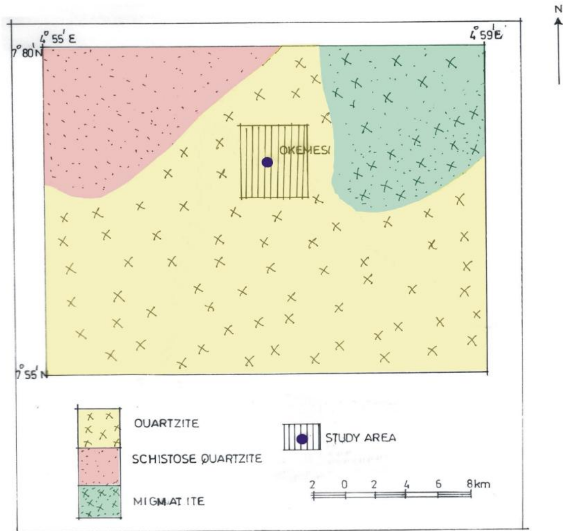
Fig. 4: Geologic map of Okemesi Ekiti
